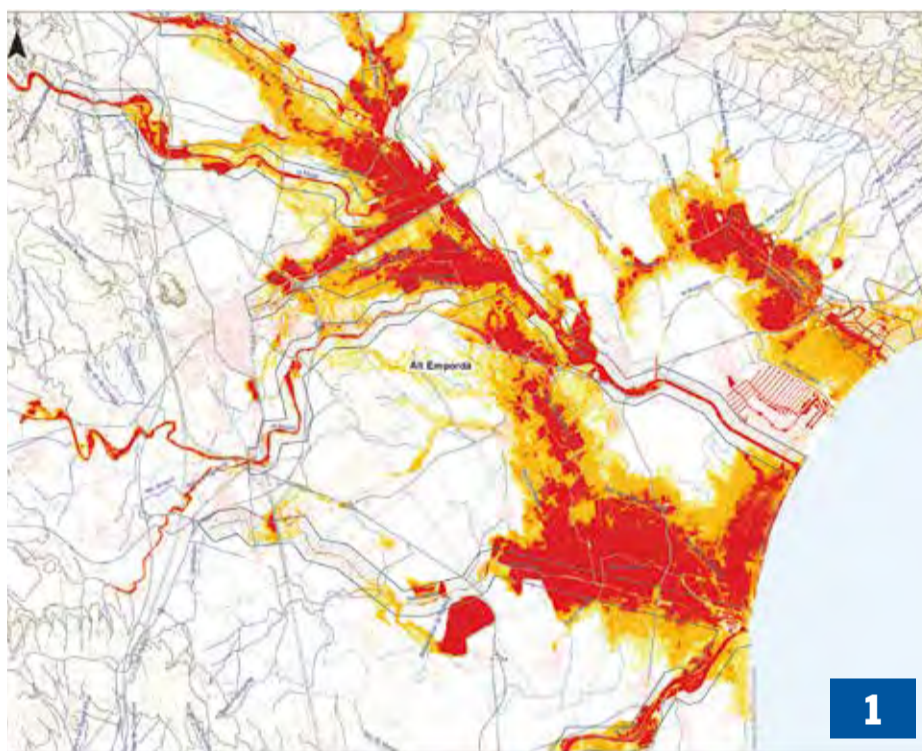
MAPES DE PERILLOSITAT PER A UN PERÍODE DE RETORN DE 100 ANYS
