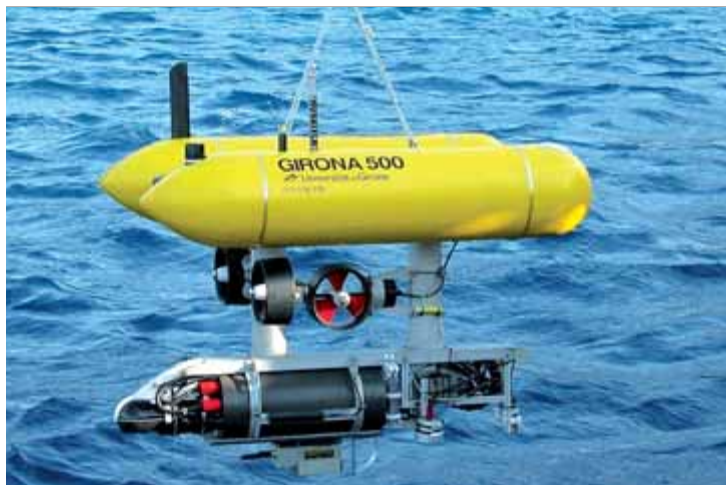
El prototip Girona 500 construït per l'equip de robòtica de la UdG ha participat en el projecte Caldera 2012, a Santorí ■ EL PUNT AVUI
