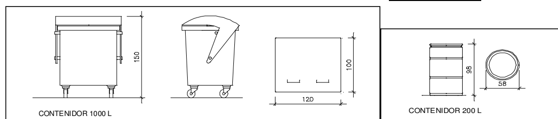
CONTENIDOR 1000 L
