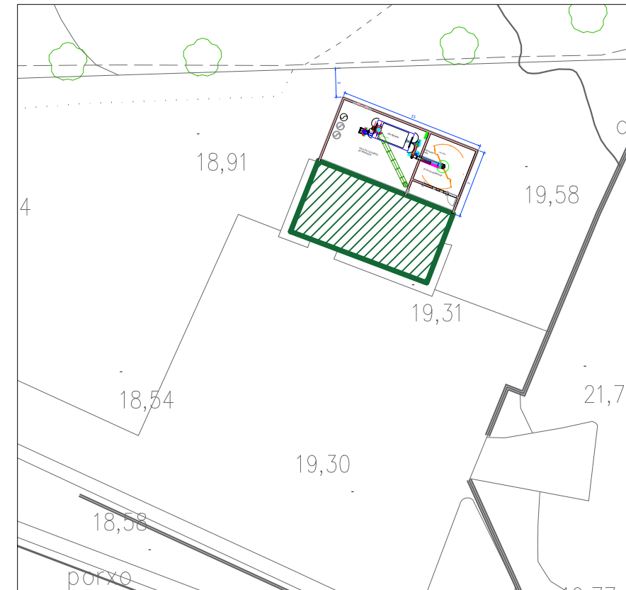
Situació sala de calderes E: 1/--
